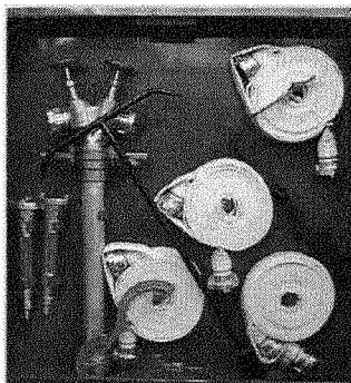
Sl. 1 Oprema podzemnog hidranta
